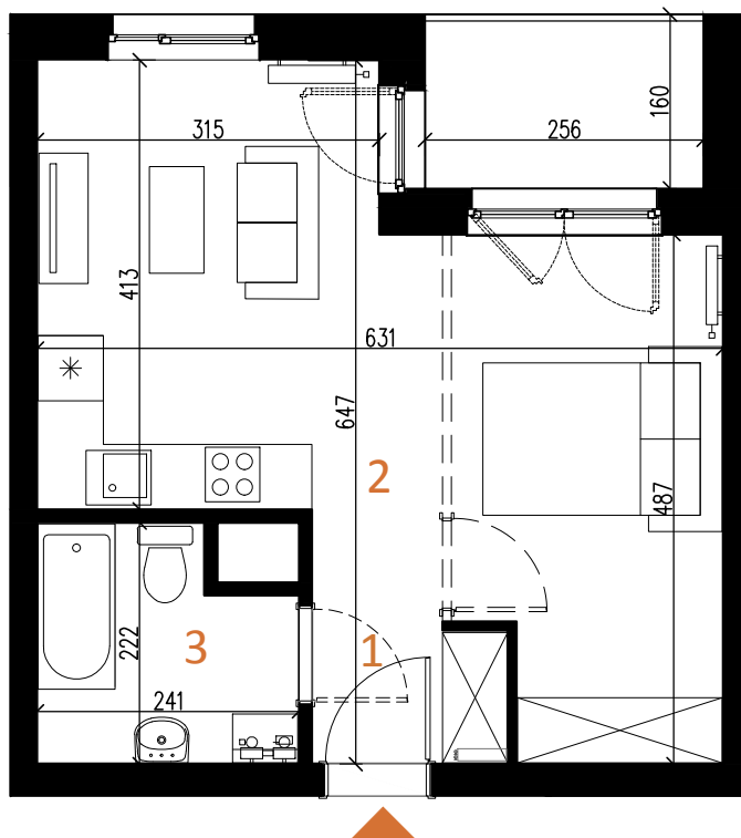
Rzut piętra
