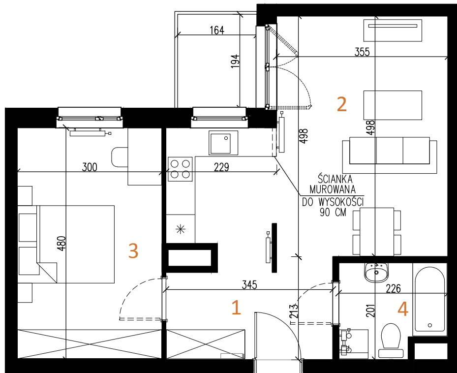
Rzut piętra
